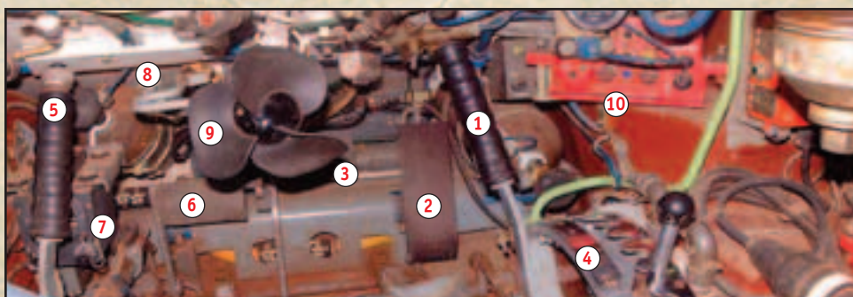
1. Рычаг управления 2. Педаль подачи топлива 3. Педаль тормоза 4. Избиратель переключения передач 5. Кнопка включения тормоза 6. Педаль сцепления 7. Гироскоп 8. Рычаг фиксатора тормоза 9. Вентилятор охлаждения (вместо конденсатора) 10. Система оповещения о пожаре
